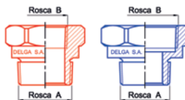
REDUCCIÓN (Rosca macho > Rosca hembra)
